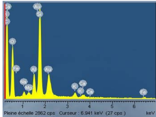
Fig. 4. Raw bentonite
