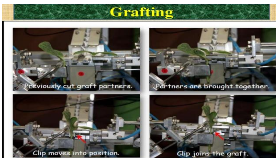
Fig. 8. Robotic grafting
